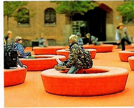
mobiliário urbano
